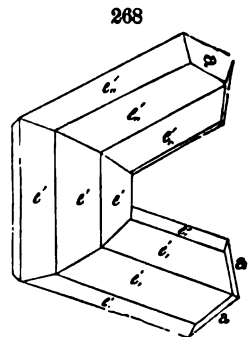
Rutile.
